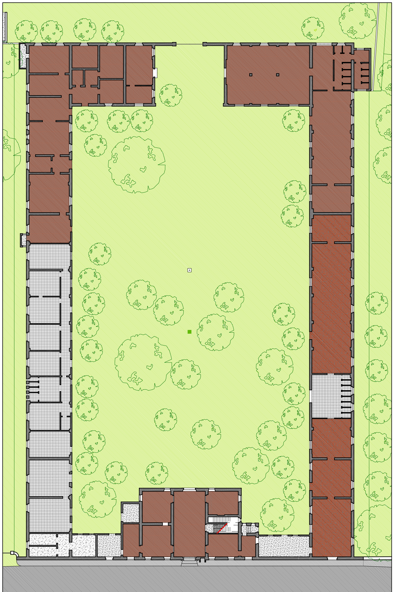
PIANTA STATO DI FATTO DELLE ALI
