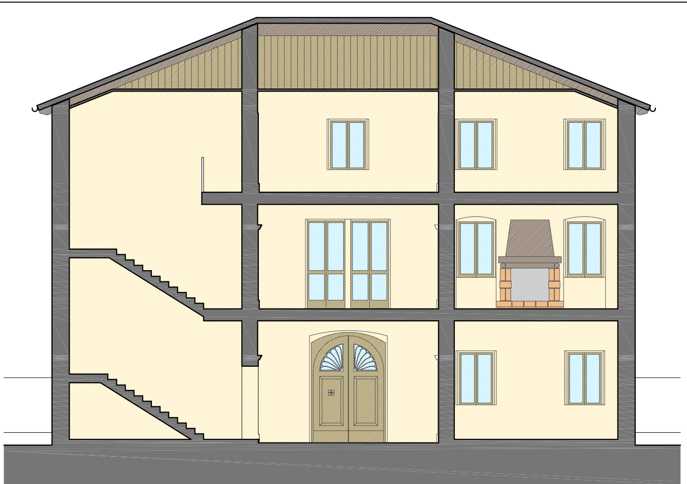
Sezione Longitudinale
